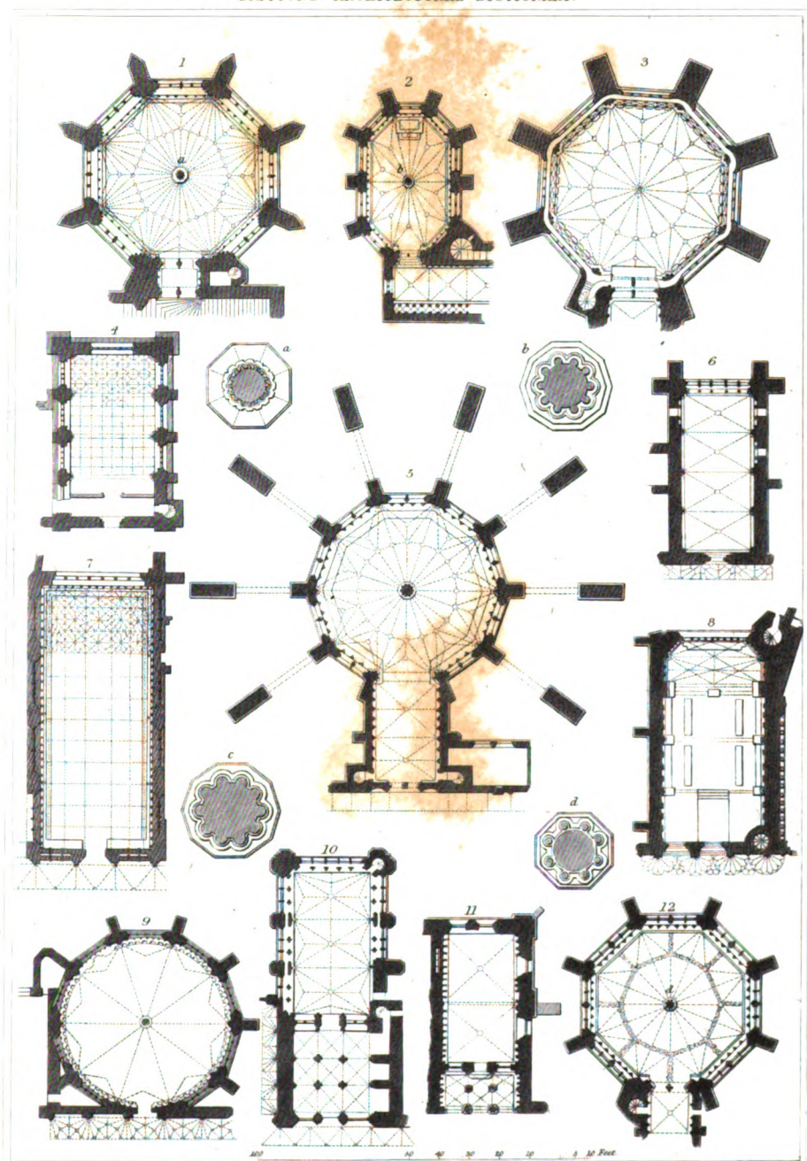
CHAPTER HOUSES.—GROUND PLANS OF 12, viz. 1. Wells.—2. Lichfield.—3. York.—4. Exeter.—5. Lincoln.—6. Durham.— 7. Canterbury.—8. Gloucester.—9. Worcester.—10. Chester.—11. Bristol.—12. Salisbury.
